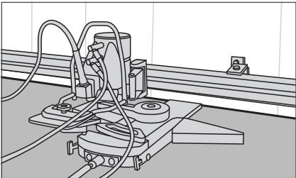
WSC 40 ermöglicht Bündigschnitten in engen Bereichen, in der Nähe von Fussboden, Decke oder Wand.
