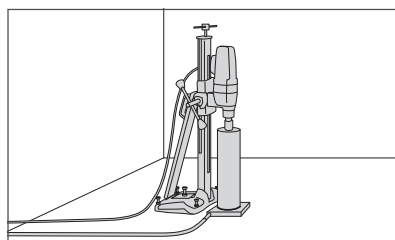
Vertikales Bohren.
